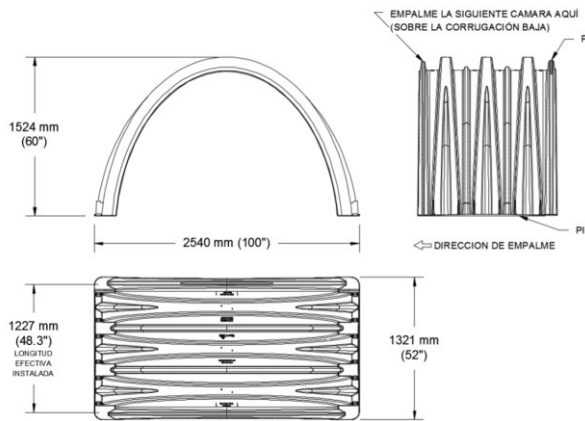
Figura 3. Dimensiones de la cámara MC-4500
