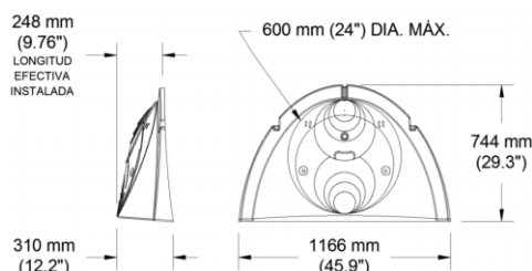
Figura 4. Dimensiones de la tapa SC-310LP / DC-780 y guías de corte.
