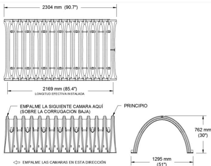
Figura 3. Dimensiones de la cámara SC-740LP
